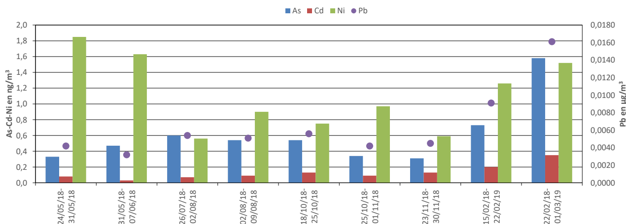
Evolution des concentrations moyennes hebdomadaires en métaux lourds des 12 derniers mois sur le site de Reims_BSN
