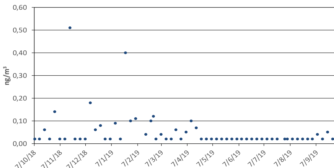
Evolution des concentrations moyennes 24h en benzo(a)pyrène des 12 derniers mois sur le site du Donon
