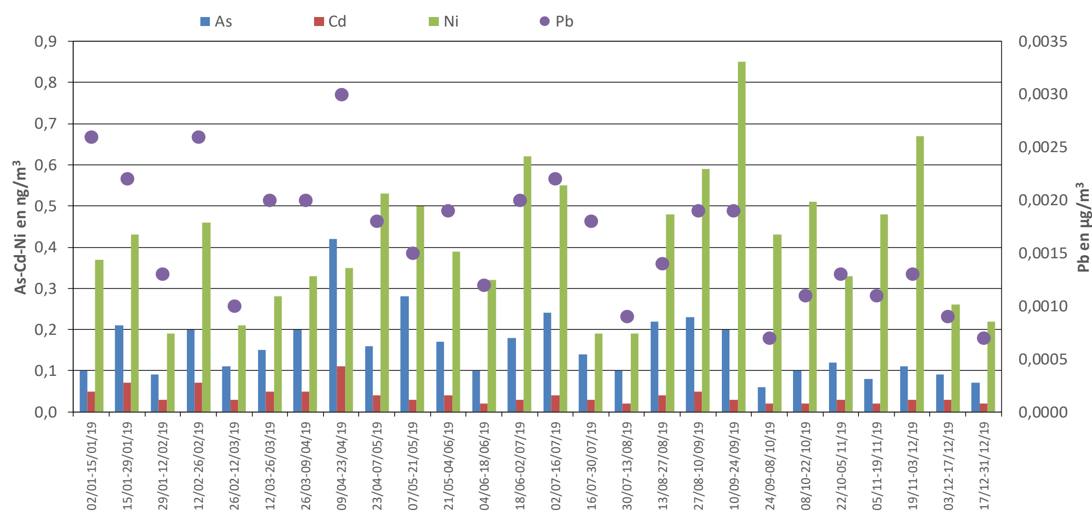
Evolution des concentrations moyennes hebdomadaires en métaux lourds des 12 derniers mois sur le site du Donon
