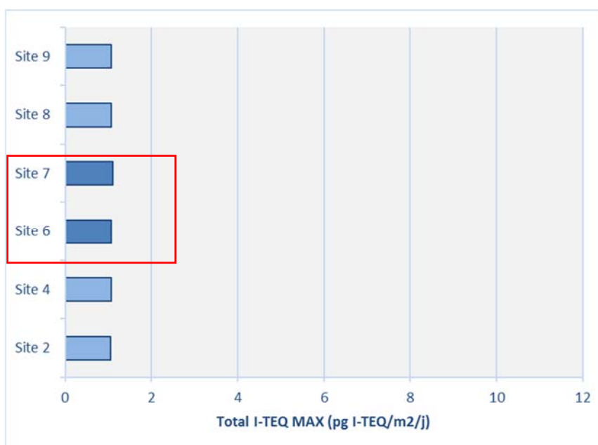
Graphique 1 : Retombées en dioxines (Total I-TEQ MAX)
