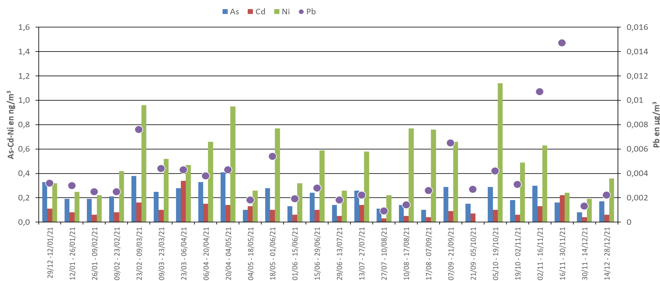
Evolution des concentrations moyennes en métaux lourds des 12 derniers mois sur le site de Revin
