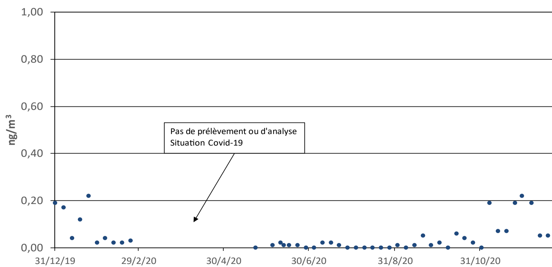
Evolution des concentrations moyennes 24h en benzo(a)pyrène des 12 derniers mois sur le site de Revin
