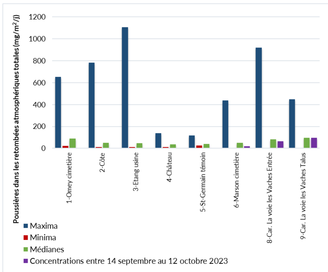
Figure 7 : Représentation graphique des retombées en poussières totales de la période analysée et comparaison aux valeurs de l'historique (2004-2023)
