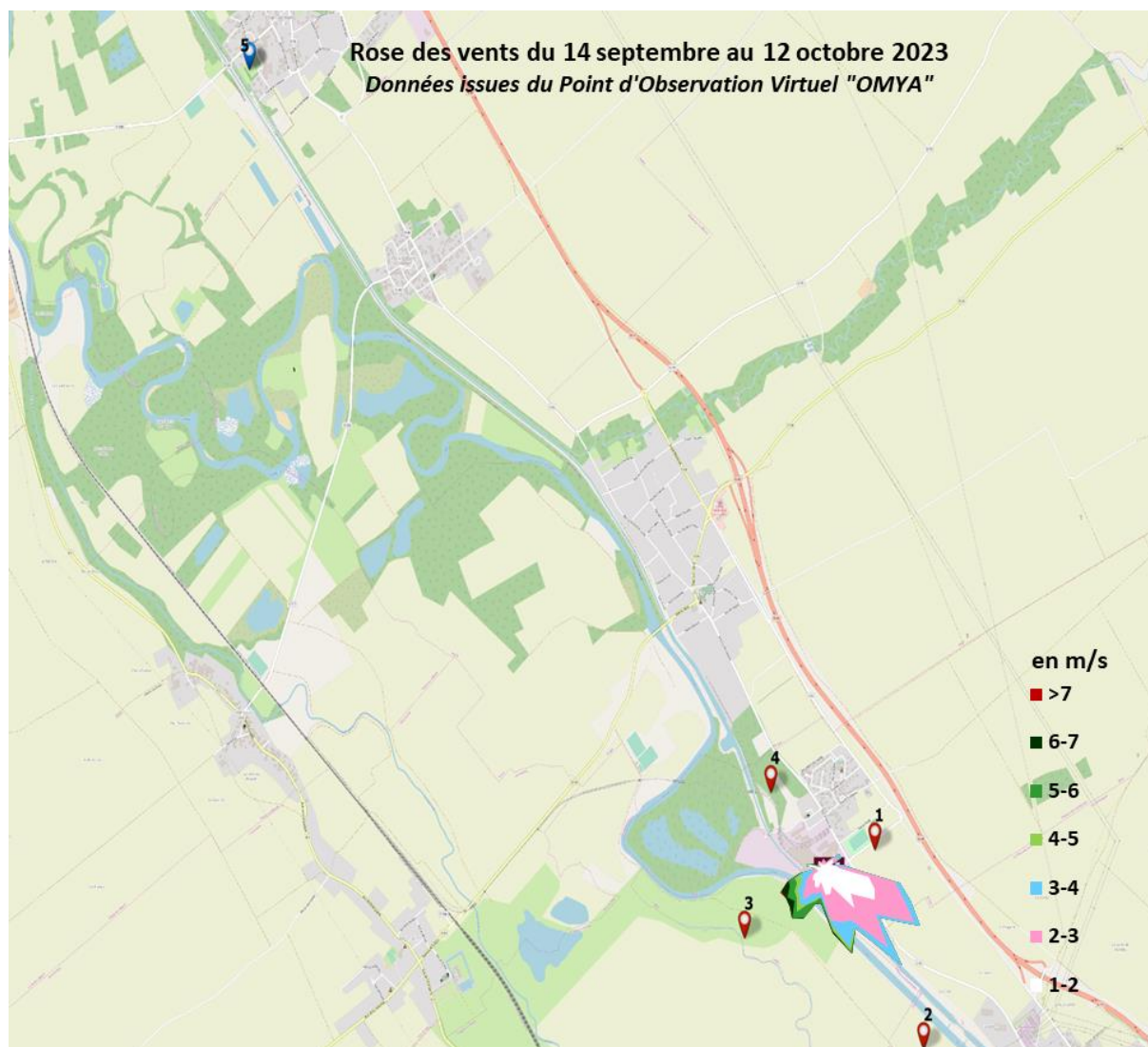
Figure 6 : Rose des vents au Point d'Observation Virtuelle « OMYA » du 14 septembre au 12 octobre 2023.
