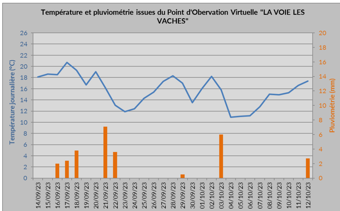
Figure 4 : Températures et précipitations journalières au point d'observation virtuelle « La Voie les Vaches » du 14 septembre au 12 octobre 2023.
