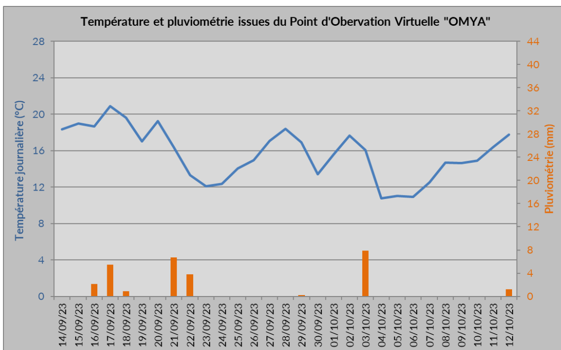
Figure 5 : Températures et précipitations journalières au point d'observation virtuelle « OMYA » du 14 septembre au 12 octobre 2023.
