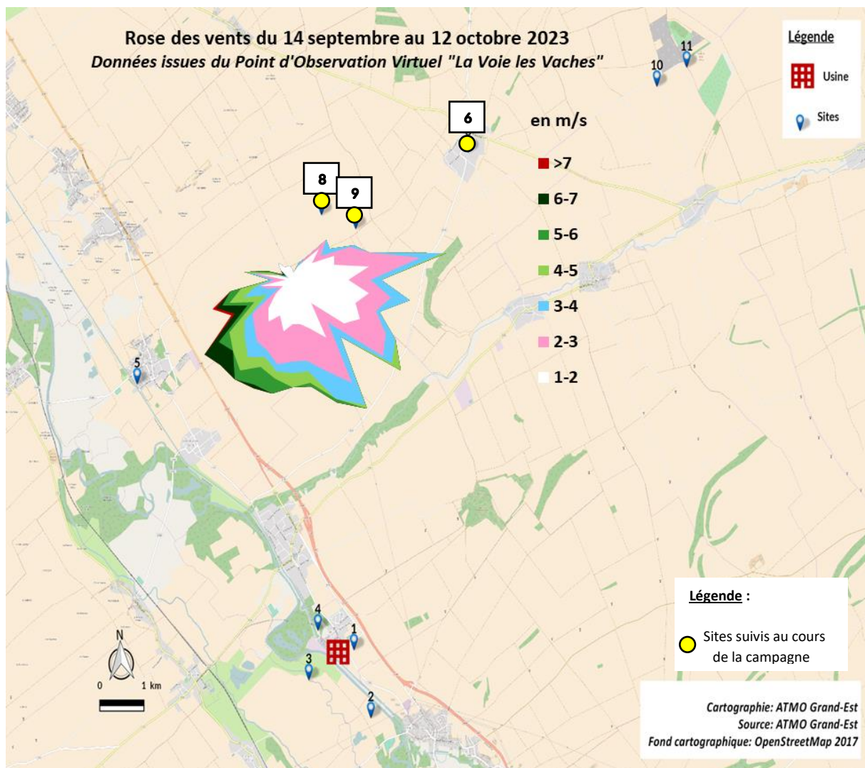
Figure 6 : Rose des vents au Point d'Observation Virtuelle « La Voie les Vaches » du 14 septembre au 12 octobre 2023.
