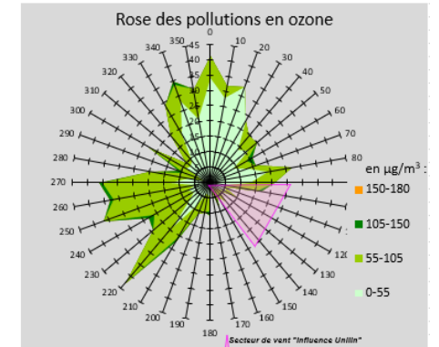
Evolution de l'ozone et rose de pollution associée
