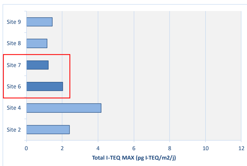
Graphique 1 : Retombées en dioxines (Total I-TEQ MAX)
