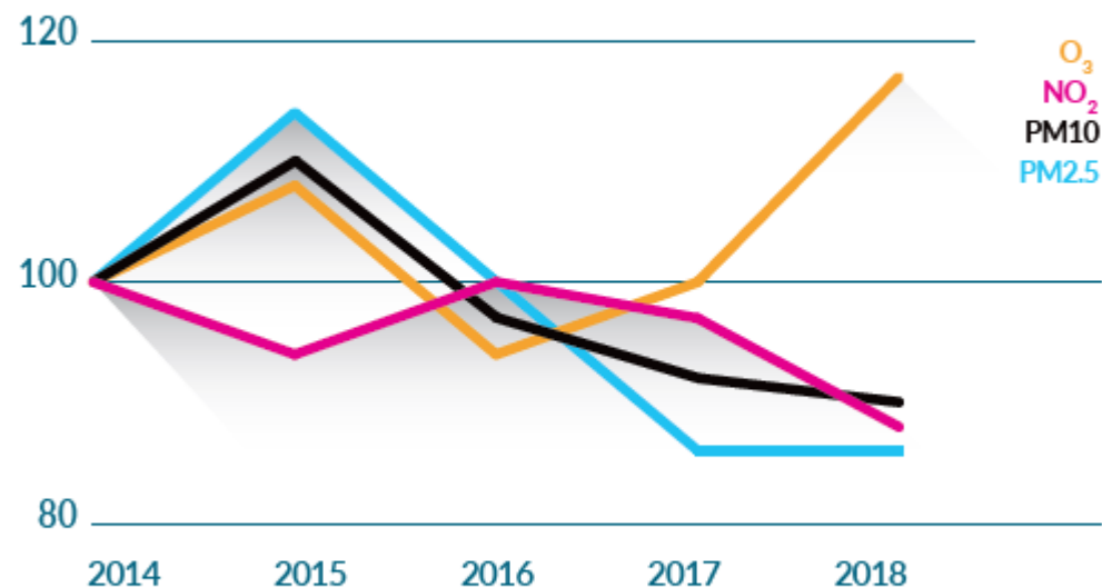
EVOLUTION DES NIVEAUX DES PRINCIPAUX POLLUANTS DE 2014 À 2018 DANS L'AUBE
