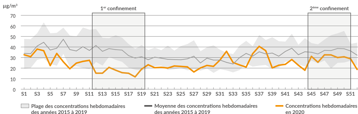
Évolution des concentrations hebdomadaires en oxydes d'azote (NO x ) dans le Grand Est en 2020 sur les sites trafics
