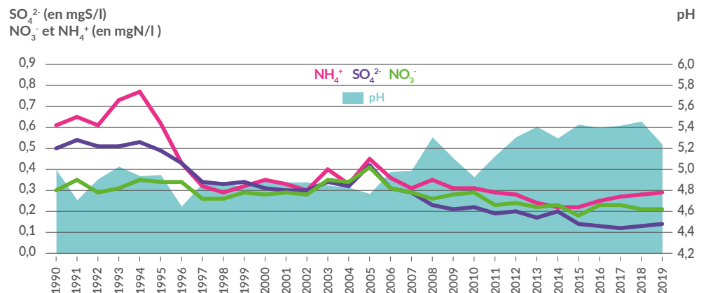
Évolution des composés soufrés ( \text{SO}_4^{2-} ) et azotés ( \text{NO}_3^- , \text{NH}_4^+ ) et du pH au Donon de 1990 à 2019
