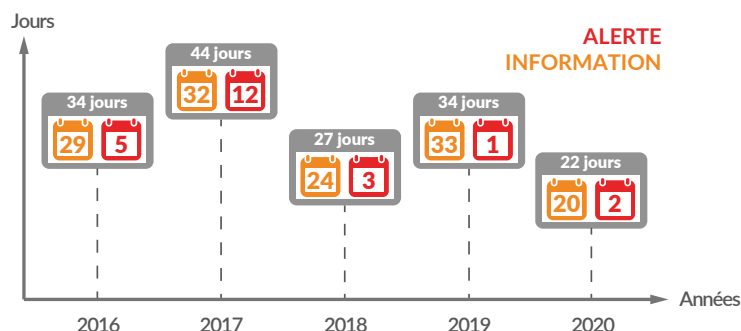
Nombre de jours de dépassement du seuil d'information-recommandations ou d'alerte pour les particules PM 10 sur les 5 dernières années
