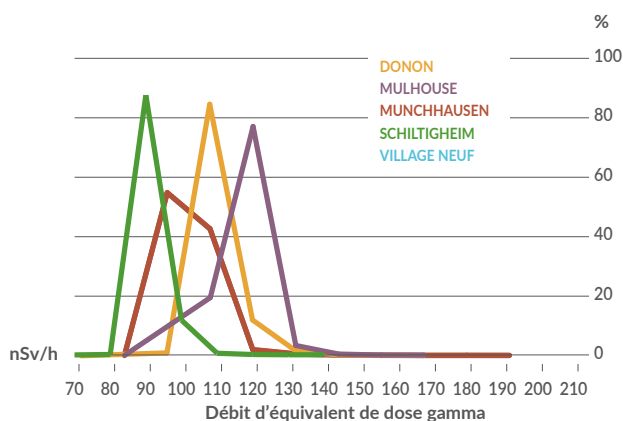
Répartition, en fréquence, du débit de dose gamma par station de mesure en 2020
