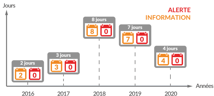
Nombre de jours de dépassement du seuil d'information-recommandations ou d'alerte pour l'ozone sur les 5 dernières années
