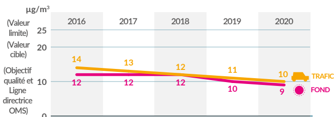
Évolution des concentrations moyennes annuelles en particules PM 2,5 selon l'influence de 2016 à 2020 (µg/m 3 )
