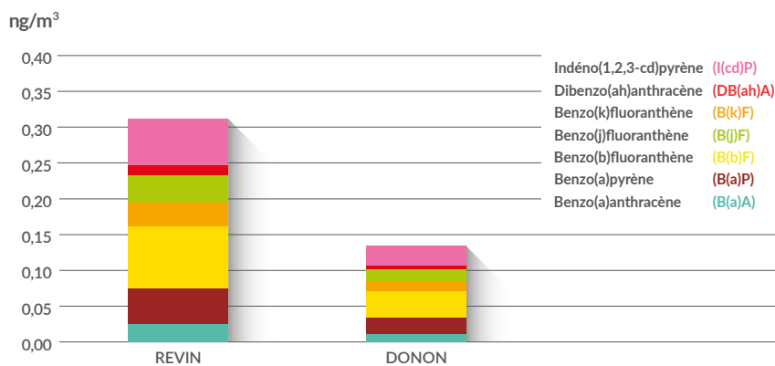
Comparaison du cumul des concentrations de HAP mesurées sur la fraction particulaire PM10 à Revin et sur le Donon en 2020
