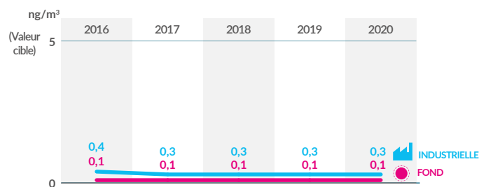
Évolution des concentrations moyennes annuelles en cadmium selon l'influence de 2016 à 2020 (ng/m³)
