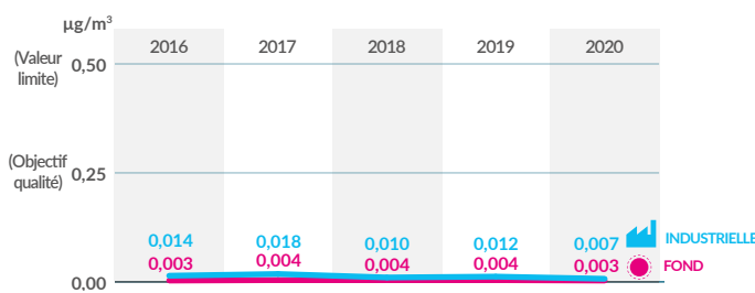
Évolution des concentrations moyennes annuelles en plomb selon l'influence de 2016 à 2020 (μg/m³)
