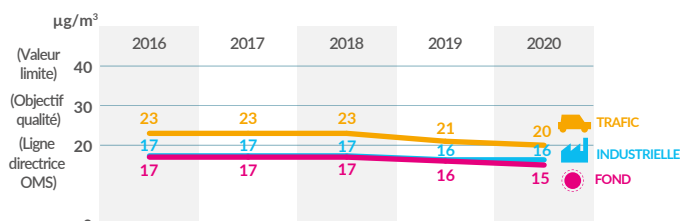
Évolution des concentrations moyennes annuelles en particules PM 10 selon l'influence de 2016 à 2020 (µg/m 3 )
