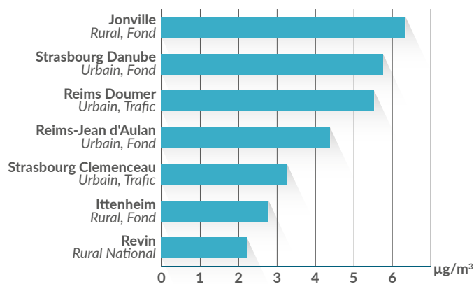
Concentrations moyennes annuelles en NH 3 en 2020
