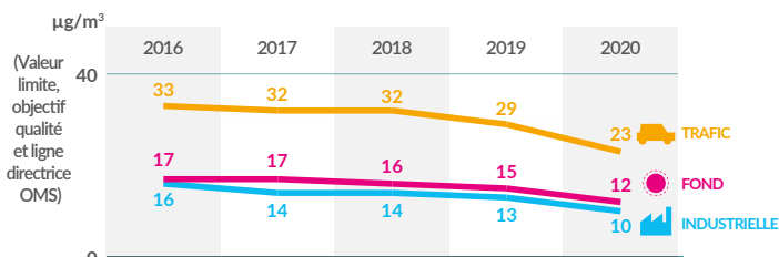
Évolution des concentrations moyennes annuelles en dioxyde d'azote selon l'influence de 2016 à 2020 ( \mu\text{g}/\text{m}^3 )
