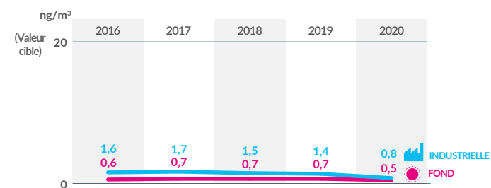
Évolution des concentrations moyennes annuelles en nickel selon l'influence de 2016 à 2020 (ng/m³)
