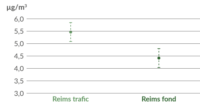
Comparaison des moyennes journalières en NH 3 sur l'agglomération de Reims sur la période janvier 2020 - février 2021
