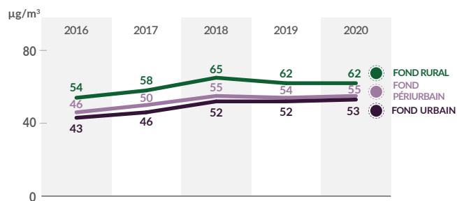
Évolution des concentrations moyennes annuelles en ozone selon l'influence de 2016 à 2020 (µg/m³)
