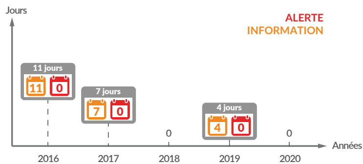
Nombre de jours de dépassement du seuil d'information-recommandations ou d'alerte pour le dioxyde d'azote sur les 5 dernières années
