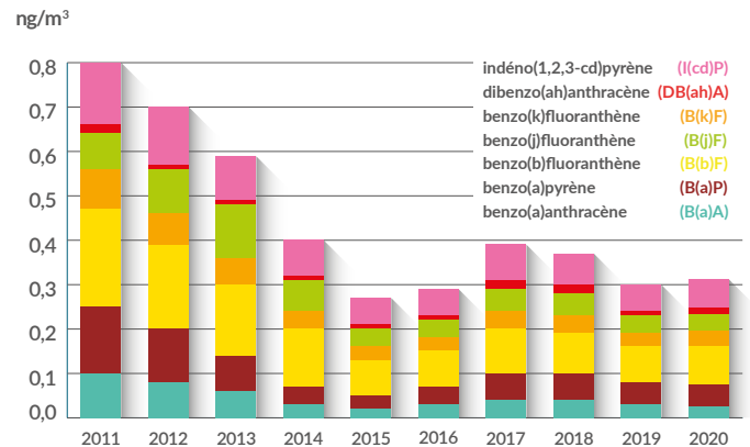
Evolution du cumul des concentrations de HAP mesurées sur la fraction particulaire PM10 à Revin de 2011 à 2020
