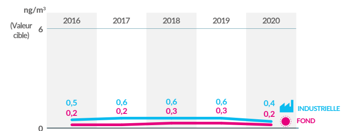
Évolution des concentrations moyennes annuelles en arsenic selon l'influence de 2016 à 2020 (ng/m³)
