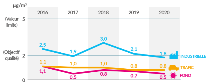
Évolution des concentrations moyennes annuelles en benzène selon l'influence de 2016 à 2020 ( \mu\text{g}/\text{m}^3 )
