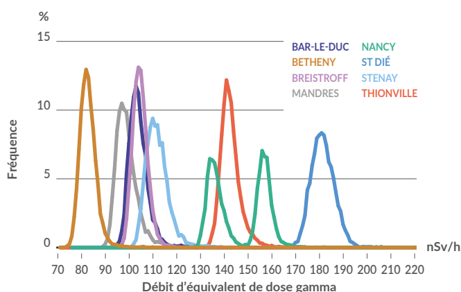
Répartition, en fréquence, du débit de dose gamma par station de mesure en 2020
