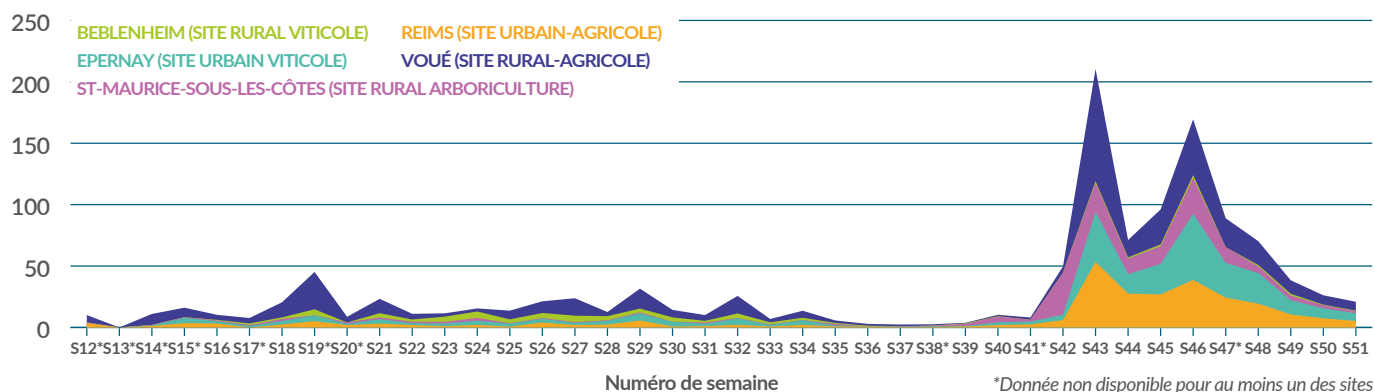
Cumul hebdomadaire des substances actives sur les sites du 16 mars au 21 décembre 2020
