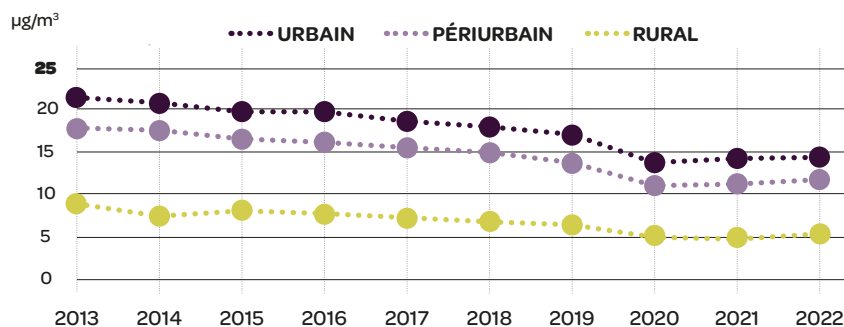
Évolution des moyennes annuelles en \text{NO}_2 en situation de fond (2013-2022)
