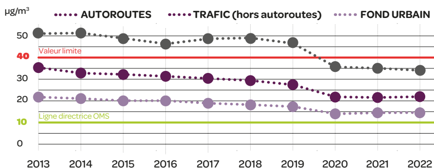
Évolution des moyennes annuelles par influence des stations en \text{NO}_2 (2013-2022)
