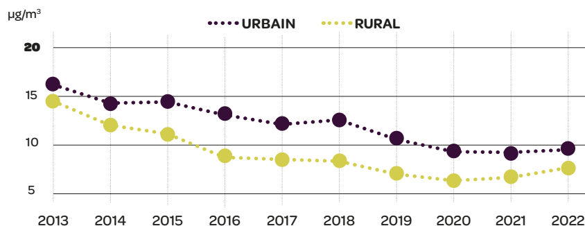
Évolution des moyennes annuelles en \text{PM}_{2,5} en situation de fond (2013-2022)
