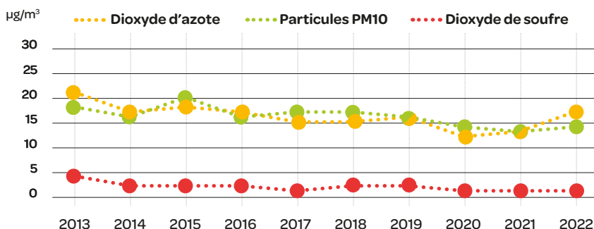
Evolution des moyennes annuelles à la station industrielle de Carling
