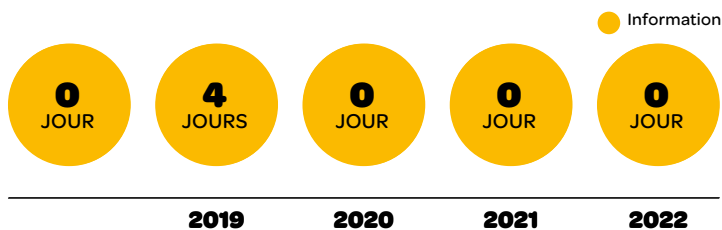
Nombre de jours de dépassement du seuil horaire de 200 \mu\text{g}/\text{m}^3 en \text{NO}_2 sur les stations d'influence trafic (autoroutes comprises)
