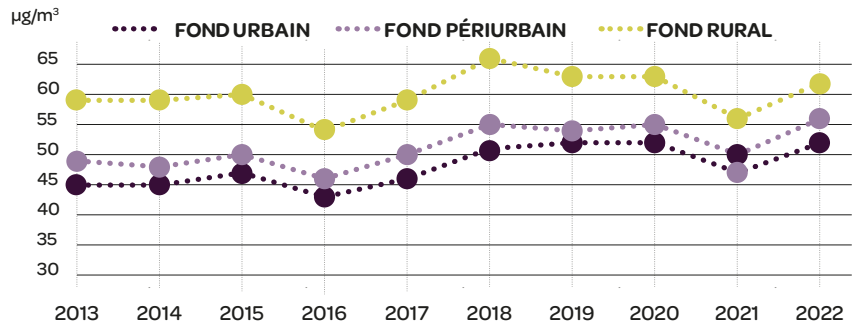
Évolution des concentrations en ozone selon la typologie de 2013 à 2022
