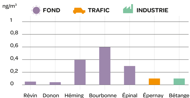
Moyennes annuelles en B(a)P dans les PM10 en 2022
