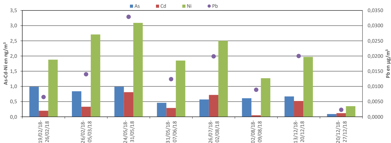
Evolution des concentrations moyennes hebdomadaires en métaux lourds des 12 derniers mois sur le site de Neuves-Maisons
