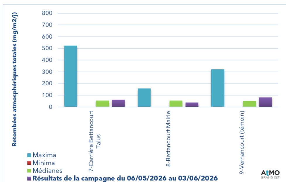
Figure 7 : Représentation graphique des retombées atmosphériques totales en poussières de la période analysée et comparaison aux valeurs de l'historique (2004-2026) pour les sites autour de la carrière Bettancourt.
