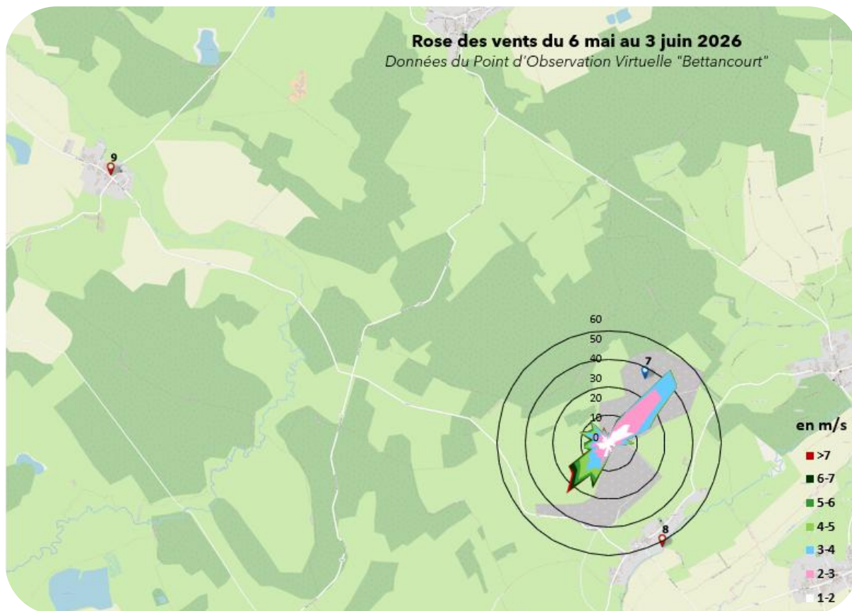
Figure 5 : Rose des vents au point d'observation virtuelle « Couvrot ».
